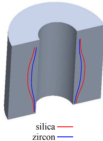
(d) Final inner diameter profile
