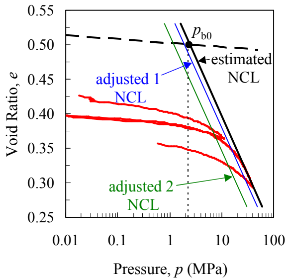
(d) Shifted Normal Consolidation Lines
